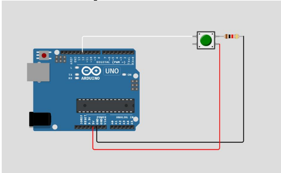
Figura 2 – Circuito Botão Interno
