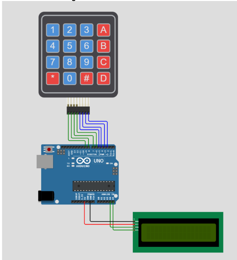
Figura 1 – Circuito Interface Usuário
